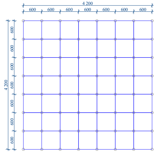
POKLÁDKA NA TERČE S DLAŽBOU FORMÁTU 120X60 CM PRŮMĚRNÁ SPOTŘEBA TERČŮ 3,57 KS/M 2
