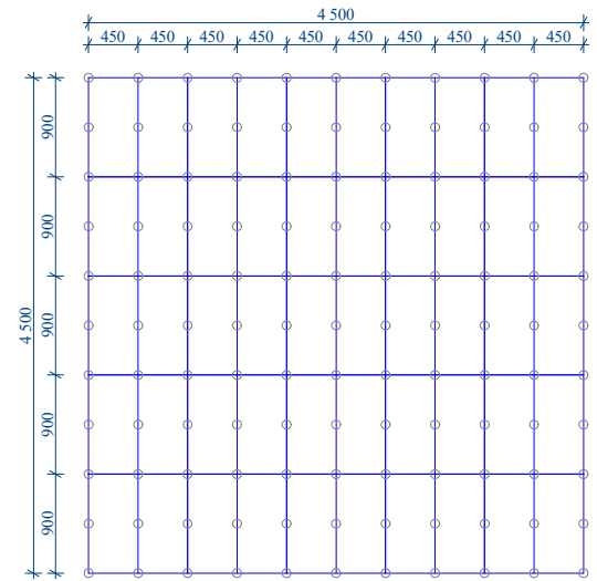
POKLÁDKA NA TERČE S DLAŽBOU FORMÁTU 90X45 CM PRŮMĚRNÁ SPOTŘEBA TERČŮ 5,98 KS/M 2
